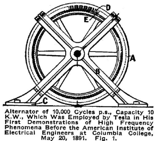
(Nikola Tesla が作った交流発電機。1891 年に実地作動された。)
